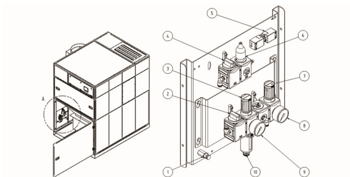
Fig. 10: Unidad de aire comprimido
